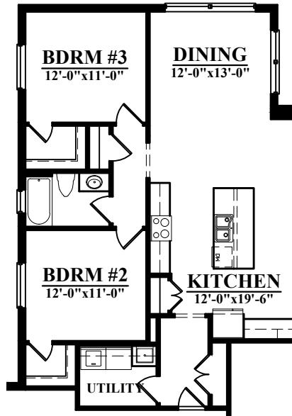
3 BEDROOM OPTION MINUS 267 S.F.
